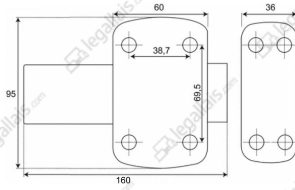
Pêne rallongé
