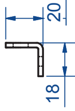
Equerre 1 trou
